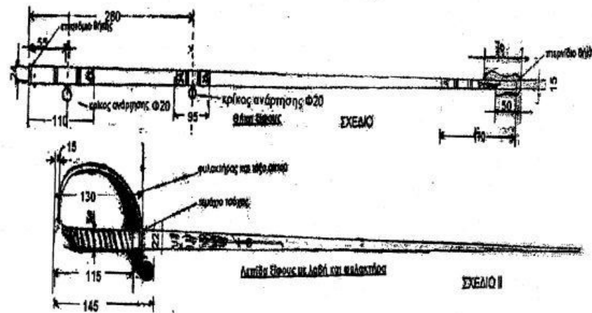
ΣΧΕΔΙΟ ΞΙΦΟΥΣ (ΓΕΝ)
