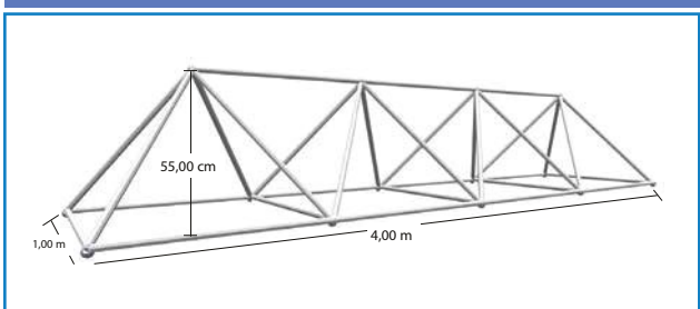
Χωροδικτύωμα
